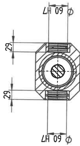
PRZEKRÓJ C-C
